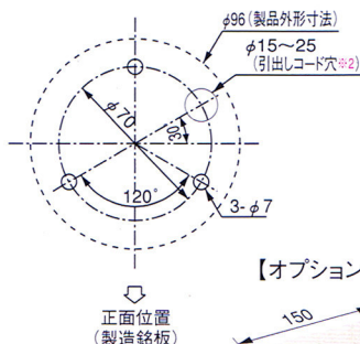
取付寸法 Mounting Dimensions
