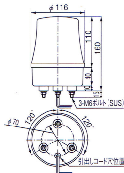
外観寸法図 Dimension
